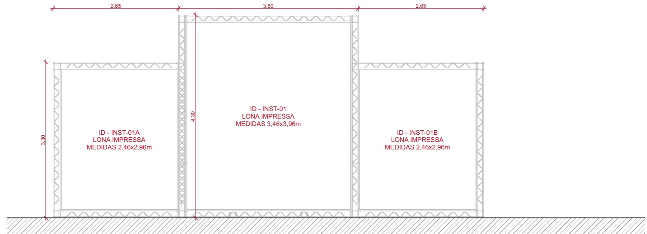
ELEVAÇÃO 01 - INSTAGRAMÁVEL 1:50
