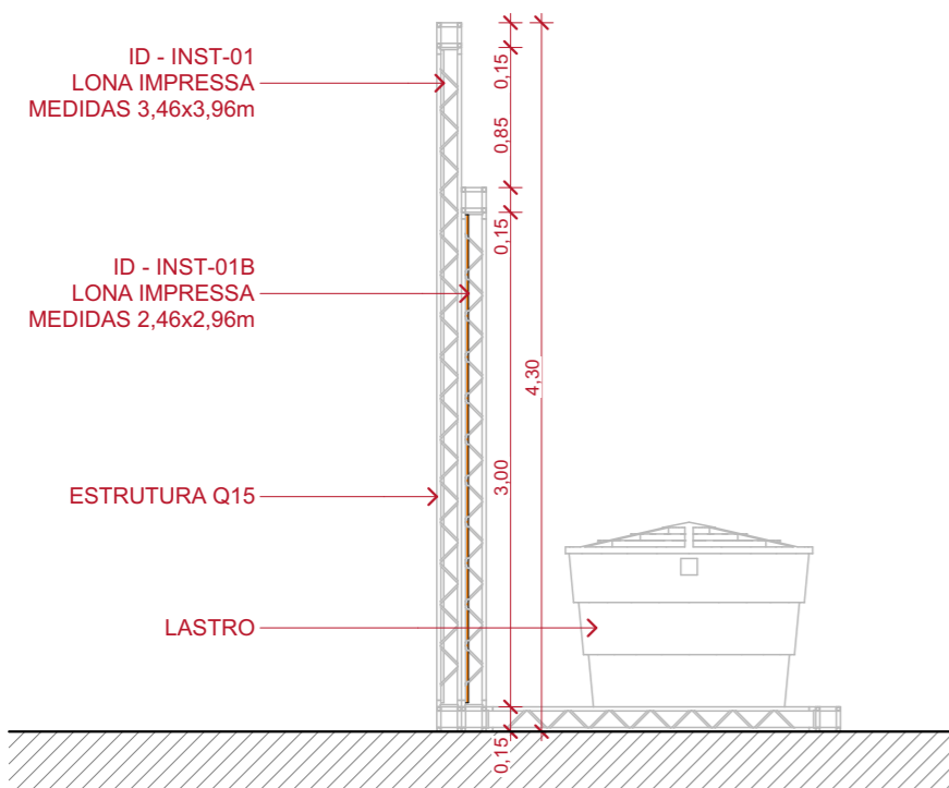
ELEVAÇÃO 02 - INSTAGRAMÁVEL 1:50
